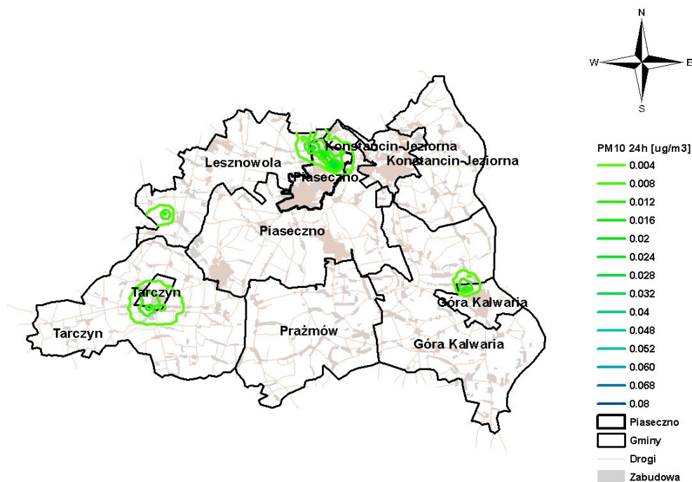
Rysunek 3.24 Rozkład stężeń pyłu zawieszono PM10 o okresie uśredniania wyników pomiarów 24 godziny pochodzących od emisji punktovej na terenie powiatu piaseczyńskiego w 2005 roku
