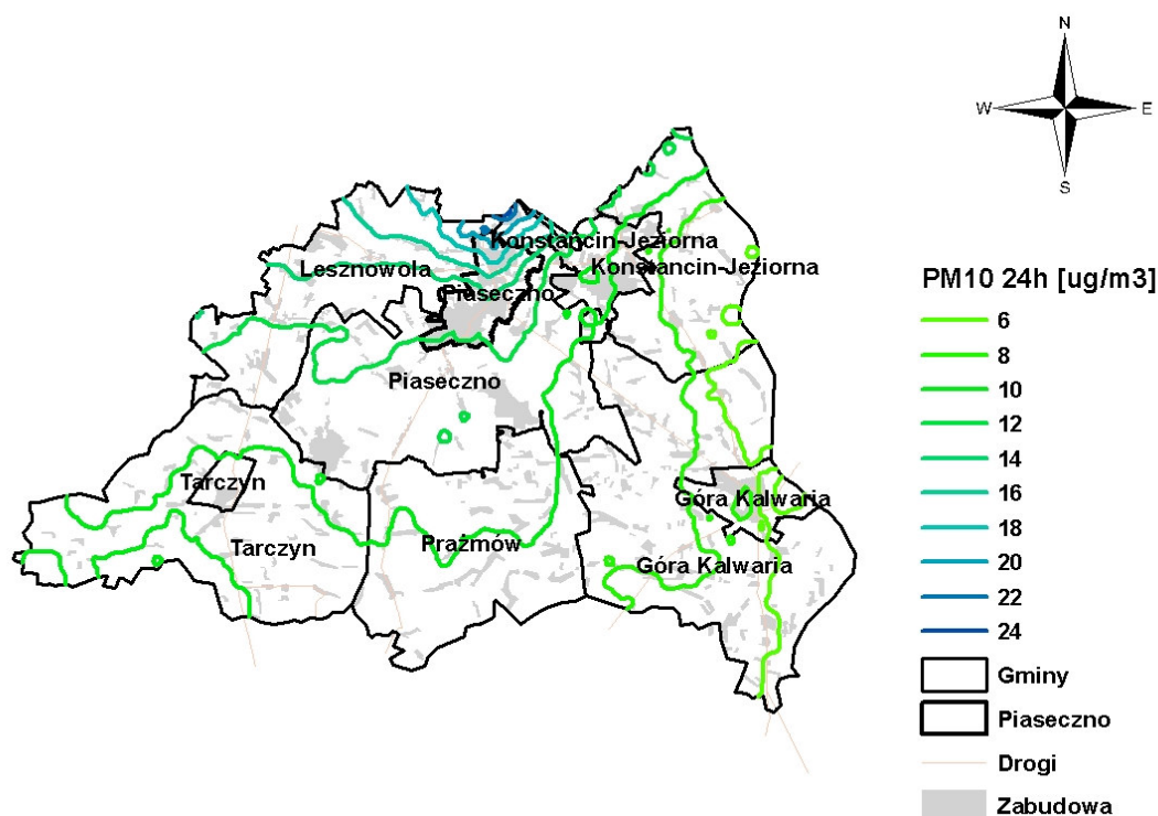
Rysunek 3.22 Stężenia pyłu zawieszonego PM10 o okresie uśredniania wyników pomiarów 24 godziny w powiecie piaseczyńskim pochodzące od emitorów liniowych zlokalizowanych w pasie 30 km od powiatu w 2005 roku
