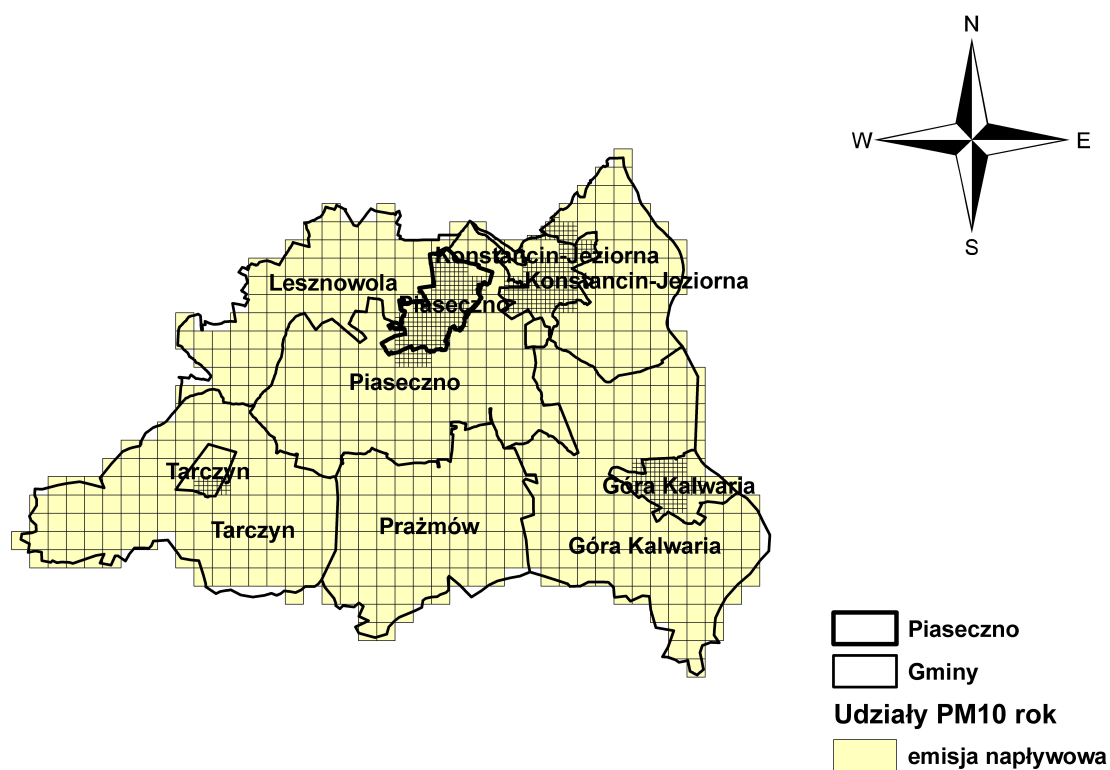
Rysunek 3.40 Udział typów emisji w imisji pyłu zawieszonego PM10 o okresie uśredniania wyników pomiarów 24 godziny w receptorach na obszarze powiatu piaseczyńskiego
