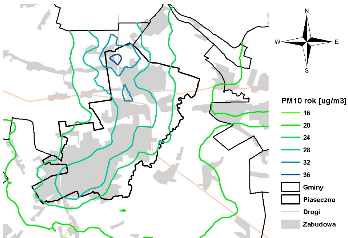
Rysunek 3.39 Rozkład stężeń pyłu zawieszonego PM10 o okresie uśredniania wyników pomiarów rok kalendarzowy w Piasecznie w 2005 roku.
