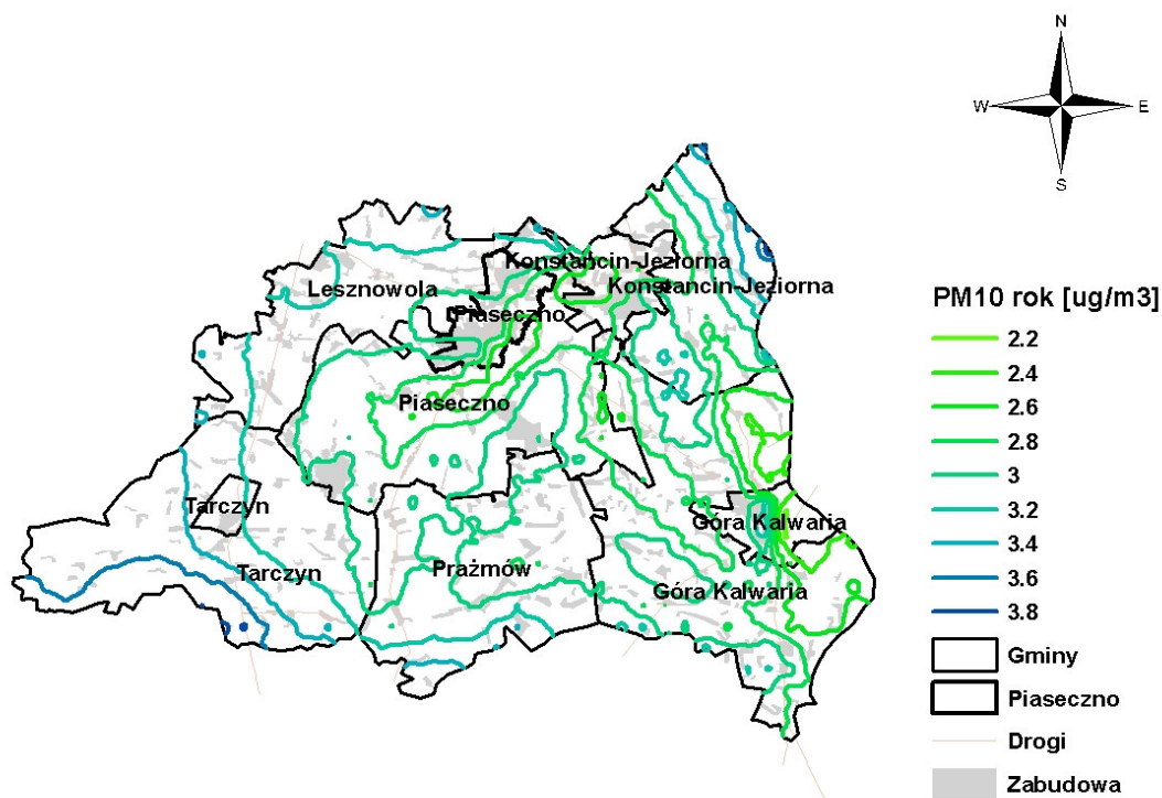
Rysunek 3.21 Stężenia pyłu zawieszonego PM10 o okresie uśredniania wyników rok kalendarzowy w powiecie piaseczyńskim pochodzące od emitorów powierzchniowych zlokalizowanych w pasie 30 km od powiatu w 2005 roku
