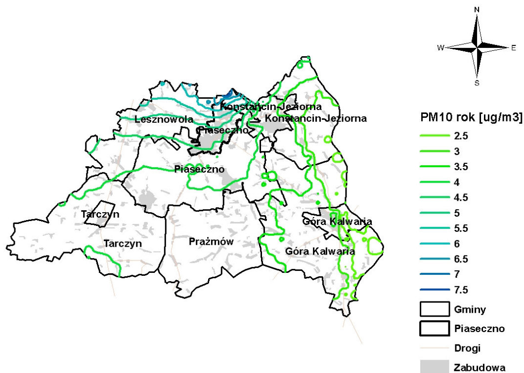
Rysunek 3.23 Stężenia pyłu zawieszonego PM10 o okresie uśredniania wyników pomiarów rok kalendarzowy w powiecie piaseczyńskim pochodzące od emitorów liniowych zlokalizowanych w pasie 30 km od powiatu w 2005 roku
