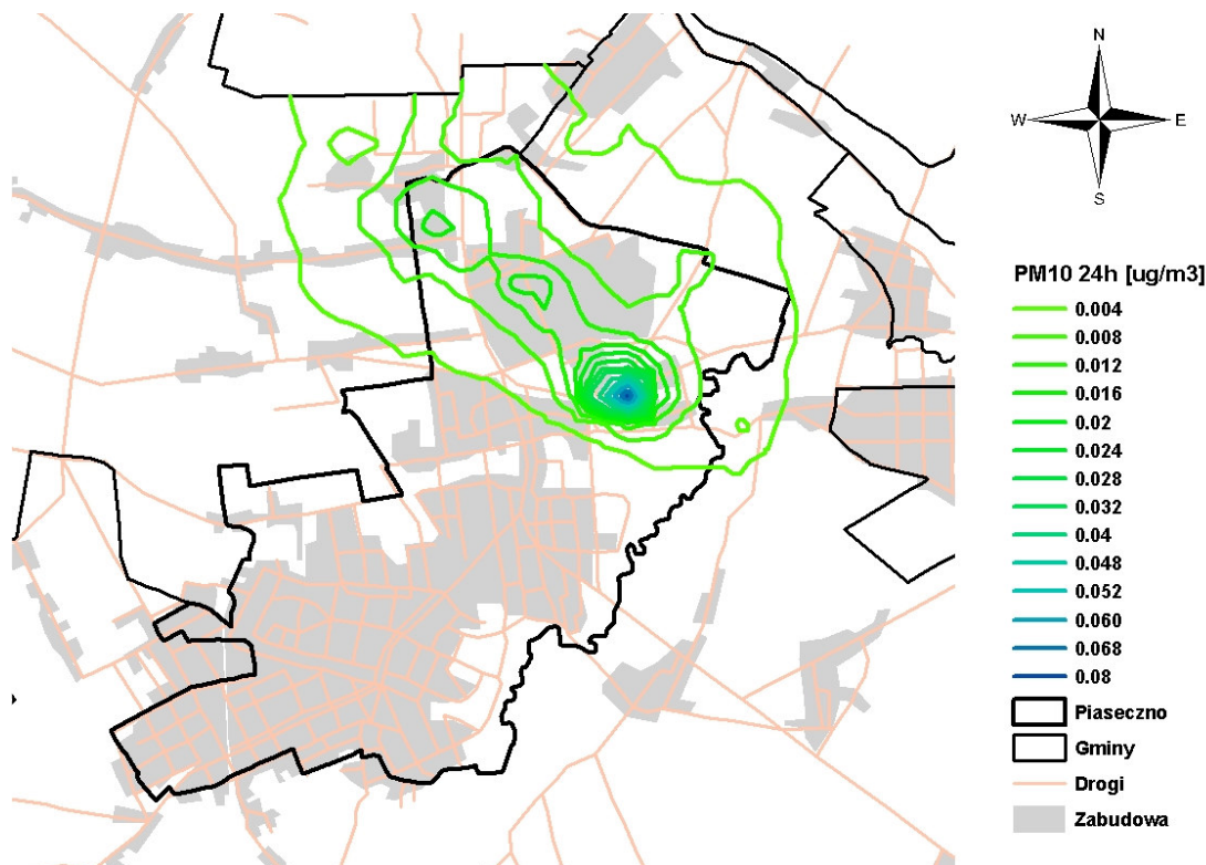
Rysunek 3.25 Rozkład stężeń pyłu zawieszono PM10 o okresie uśredniania wyników 24 godziny pochodzących od emisji punktovej w Piasecznie w 2005 roku
