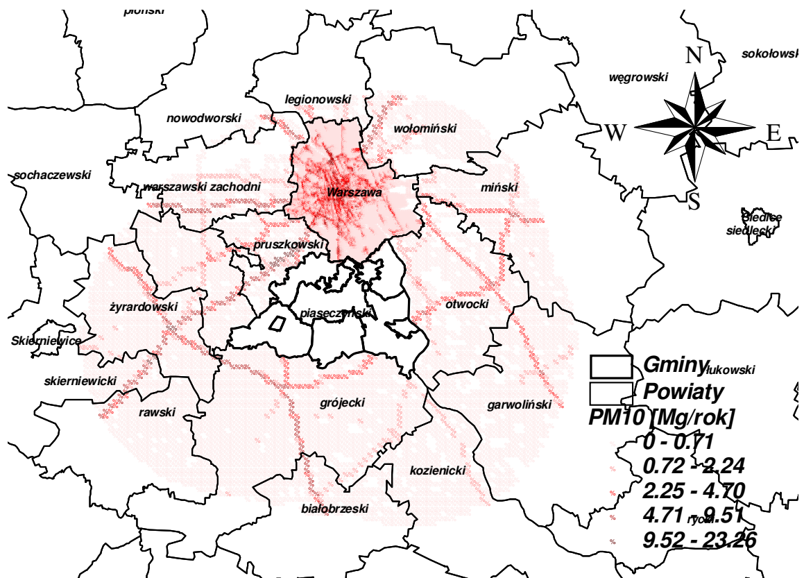
Rysunek 3.5 Całkowita emisja pyłu zawieszonego PM10 ze źródeł liniowych zlokalizowanych w pasie 30 km od powiatu piaseczyńskiego w 2005 roku
